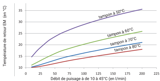
Fig. 4: Température de retour sur le circuit eau morte pour différentes températures de stockage dans le ballon tampon
