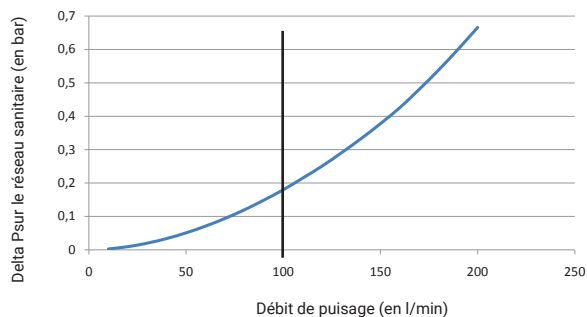
Fig. 7: Evolution des pertes de charge sur le circuit sanitaire en fonction du débit de puisage
