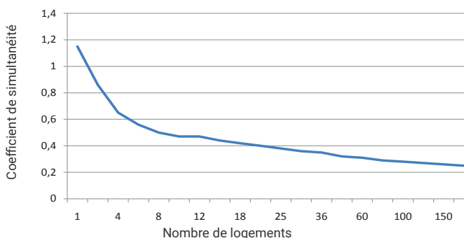
Fig. 3: Coefficient de simultanéité des puisages pour un immeuble d'habitations (3-4 personnes par logement).
