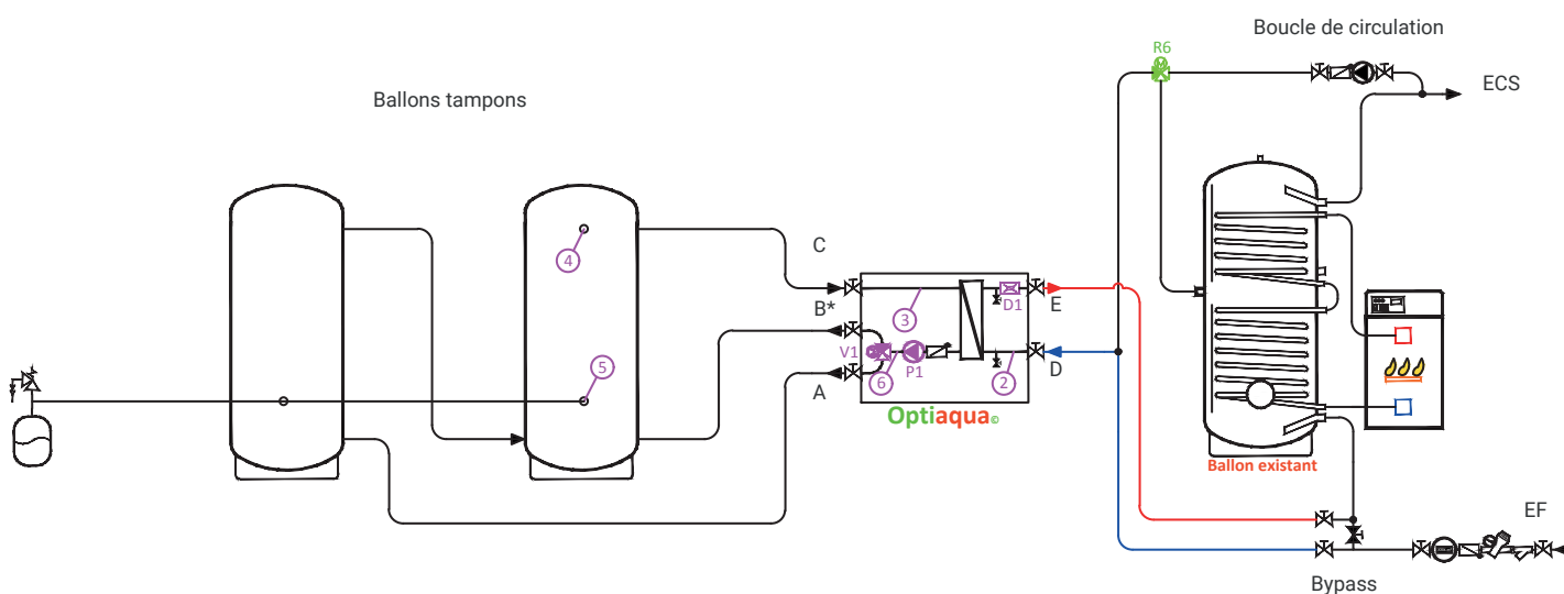
Fig. 12: Schéma hydraulique d'une installation avec stratification et boucle de circulation
