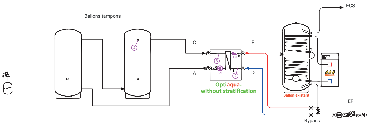
Fig. 13: Schéma hydraulique d'une installation sans stratification
