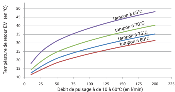
Fig. 5: Température de retour sur le circuit eau morte pour différentes températures de stockage dans le ballon tampon
