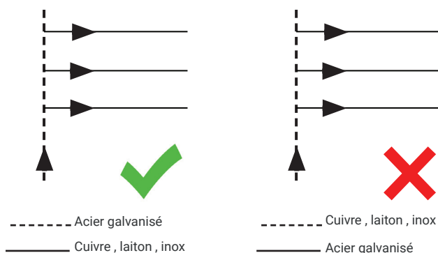
Fig. 11: Choix des matériaux en fonction de leurs positions
